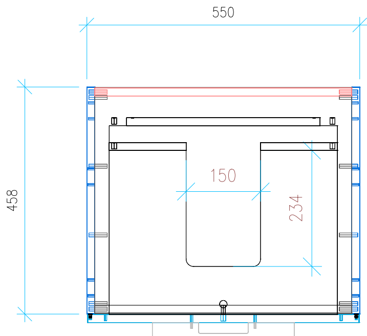
Ansicht 2 / Draufsicht
