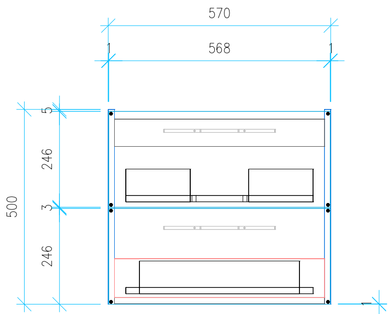
Ansicht 4 / Vorderansicht
