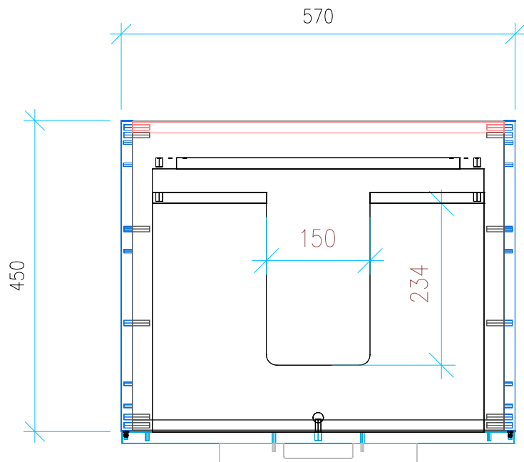
Ansicht 2 / Draufsicht
