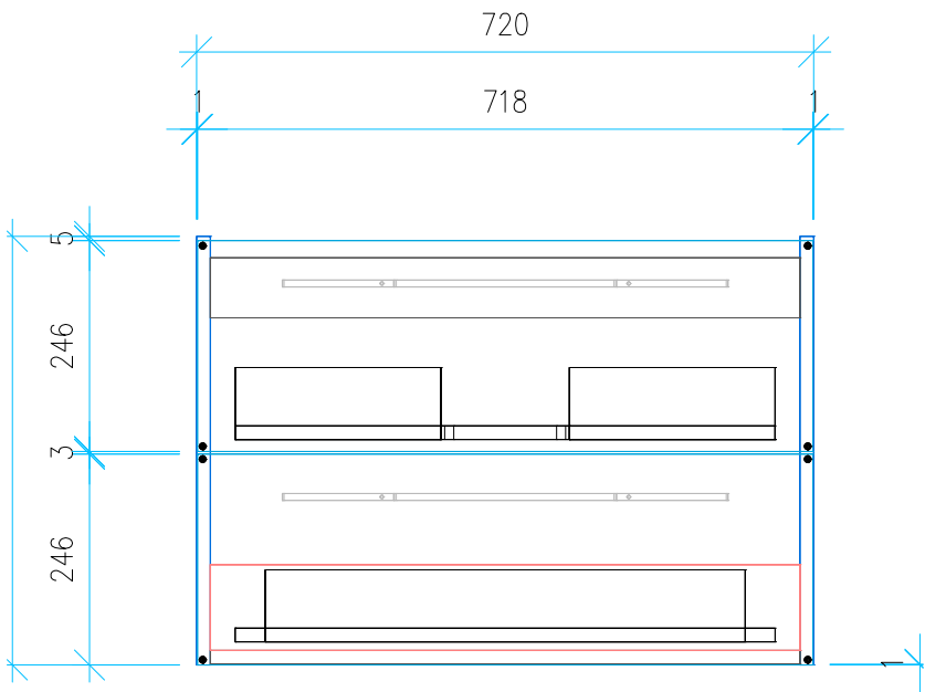
Ansicht 4 / Vorderansicht
