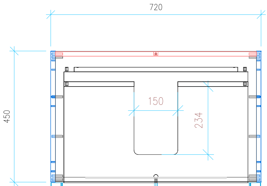
Ansicht 2 / Draufsicht
