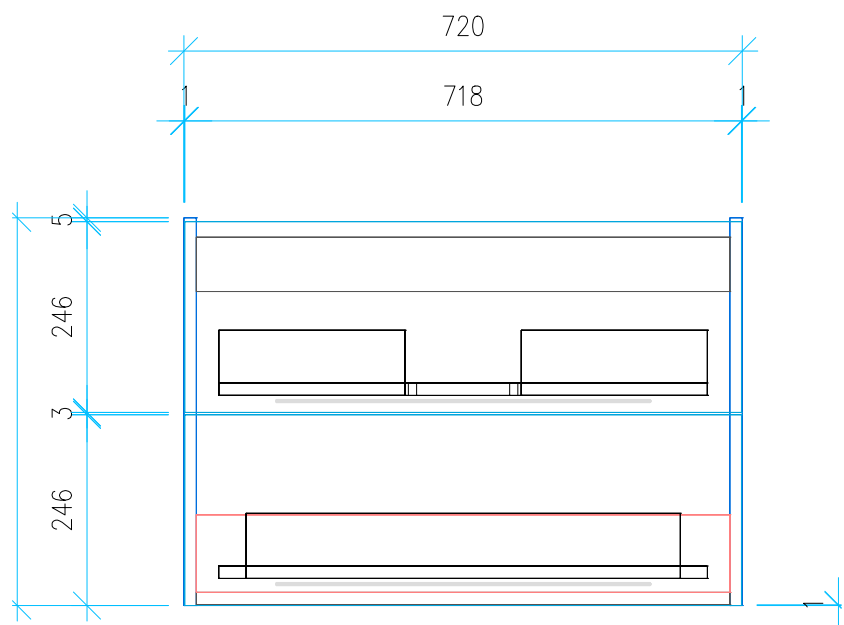
Ansicht 4 / Vorderansicht
