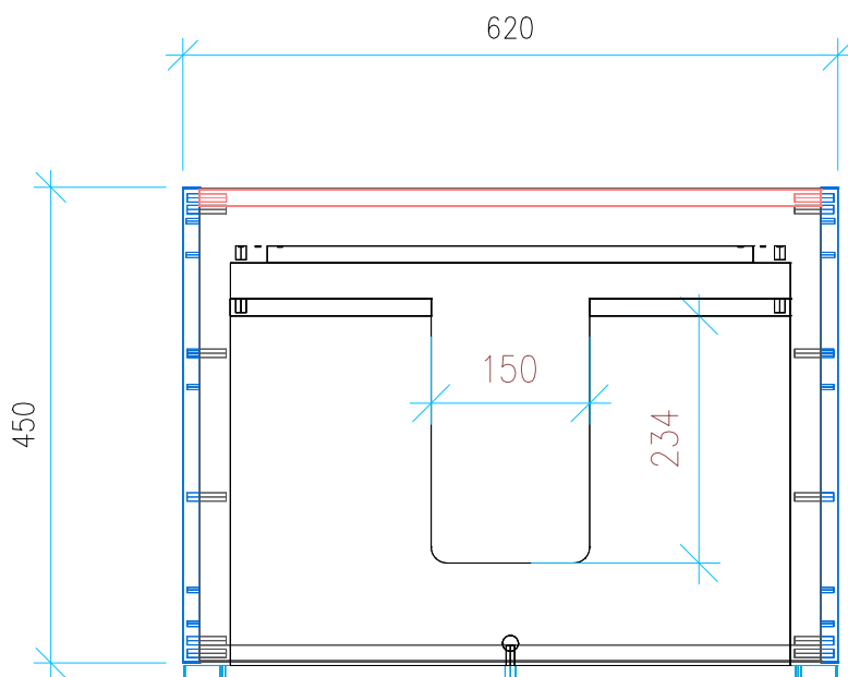
Ansicht 2 / Draufsicht
