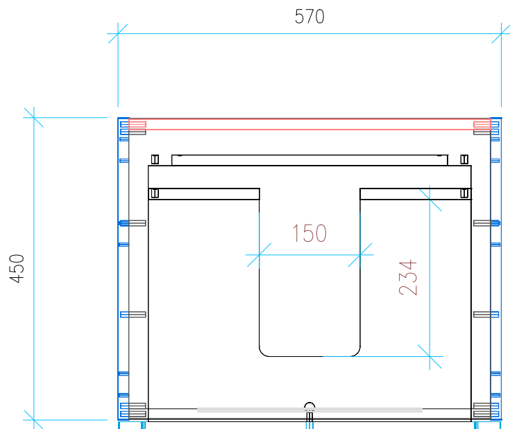
Ansicht 2 / Draufsicht
