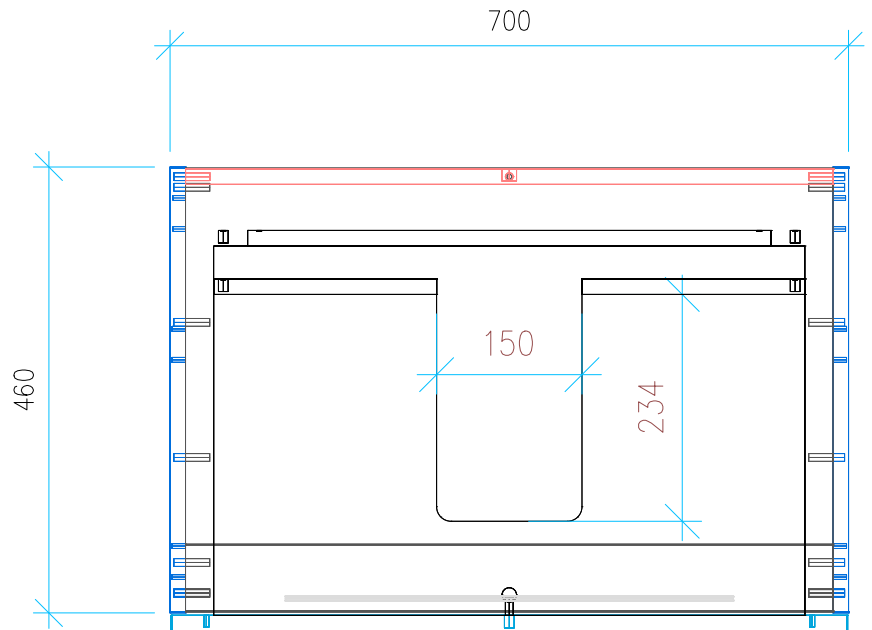
Ansicht 2 / Draufsicht
