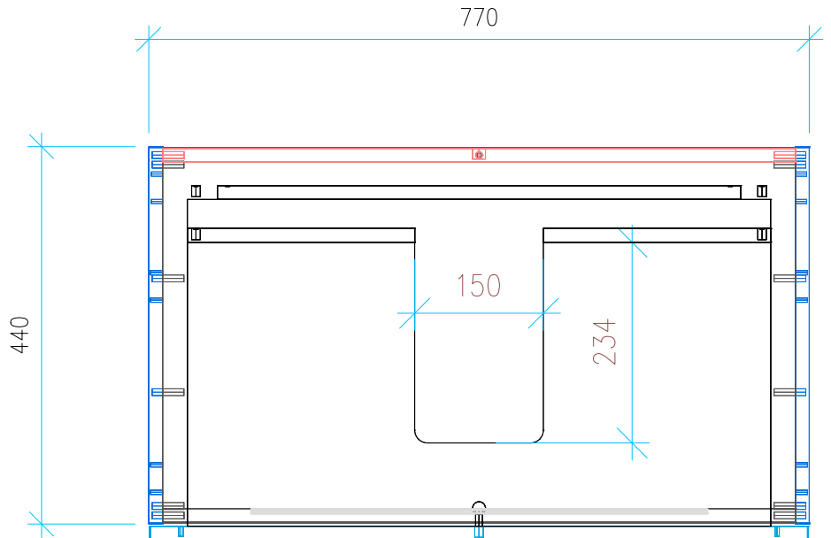
Ansicht 2 / Draufsicht
