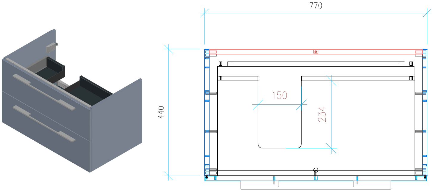
Ansicht 1 / 3D
