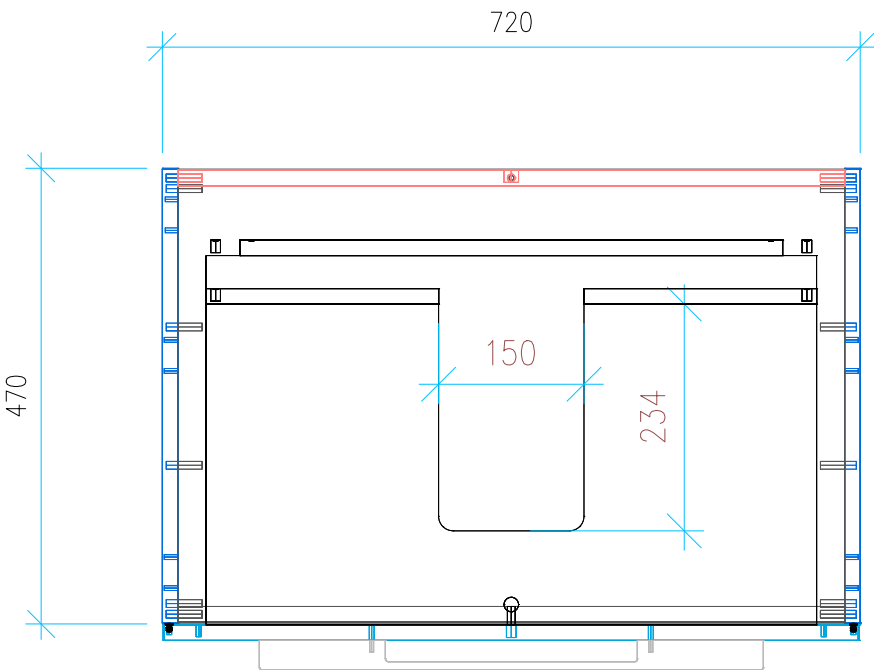
Ansicht 2 / Draufsicht
