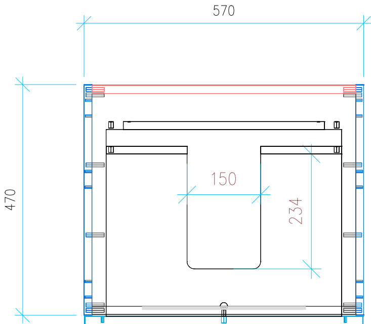
Ansicht 2 / Draufsicht
