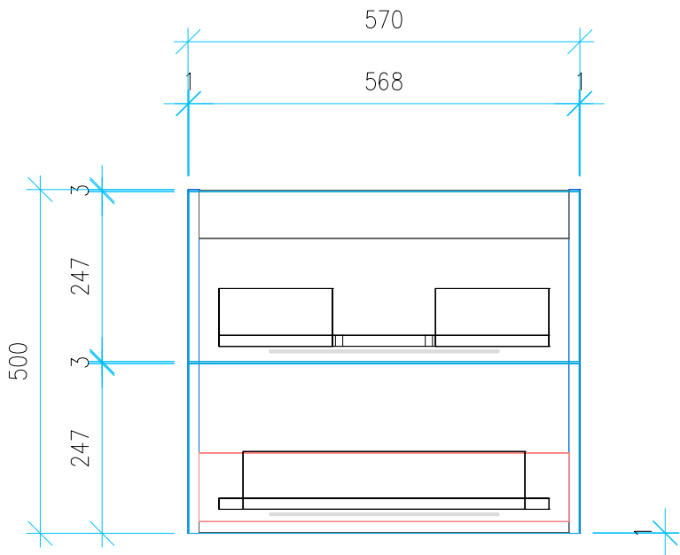
Ansicht 4 / Vorderansicht
