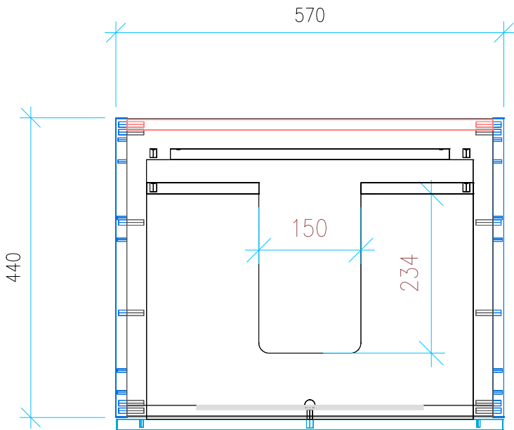
Ansicht 2 / Draufsicht
