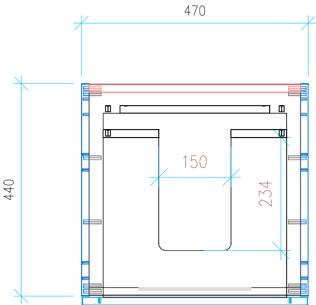
Ansicht 2 / Draufsicht
