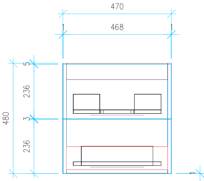
Ansicht 4 / Vorderansicht
