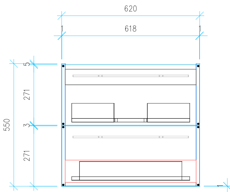
Ansicht 4 / Vorderansicht
