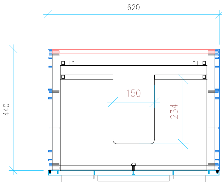
Ansicht 2 / Draufsicht
