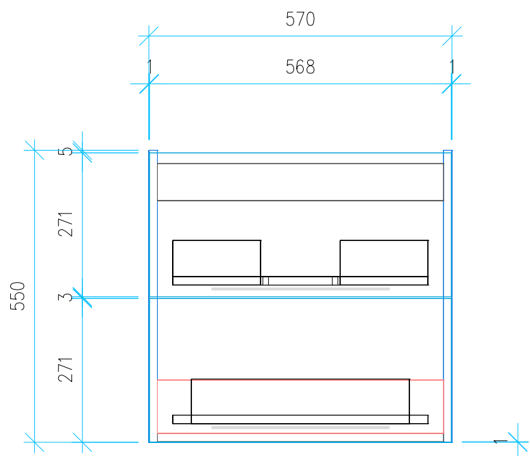
Ansicht 4 / Vorderansicht
