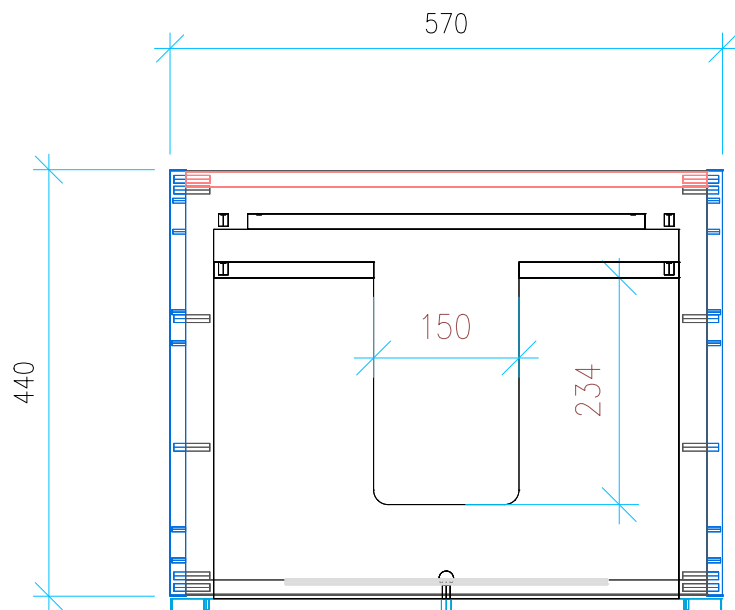
Ansicht 2 / Draufsicht
