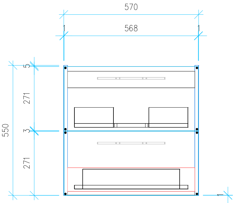
Ansicht 4 / Vorderansicht
