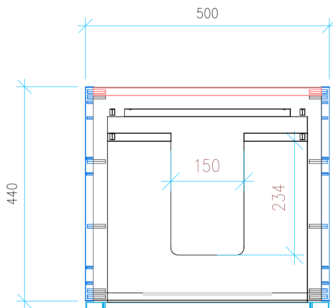
Ansicht 2 / Draufsicht
