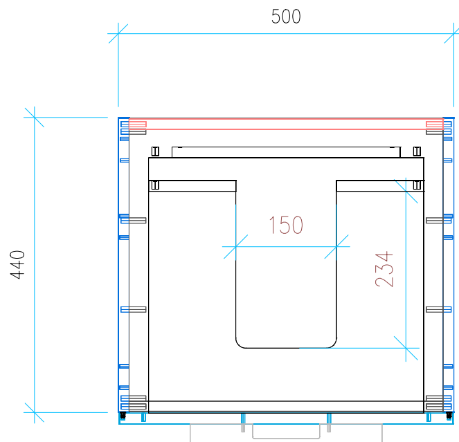
Ansicht 2 / Draufsicht
