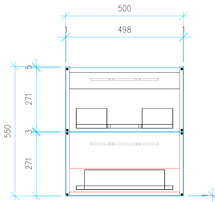
Ansicht 4 / Vorderansicht
