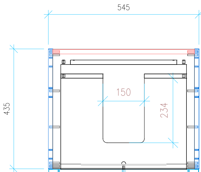
Ansicht 2 / Draufsicht
