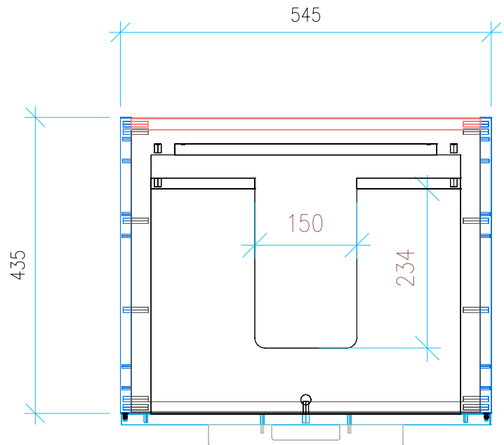
Ansicht 2 / Draufsicht
