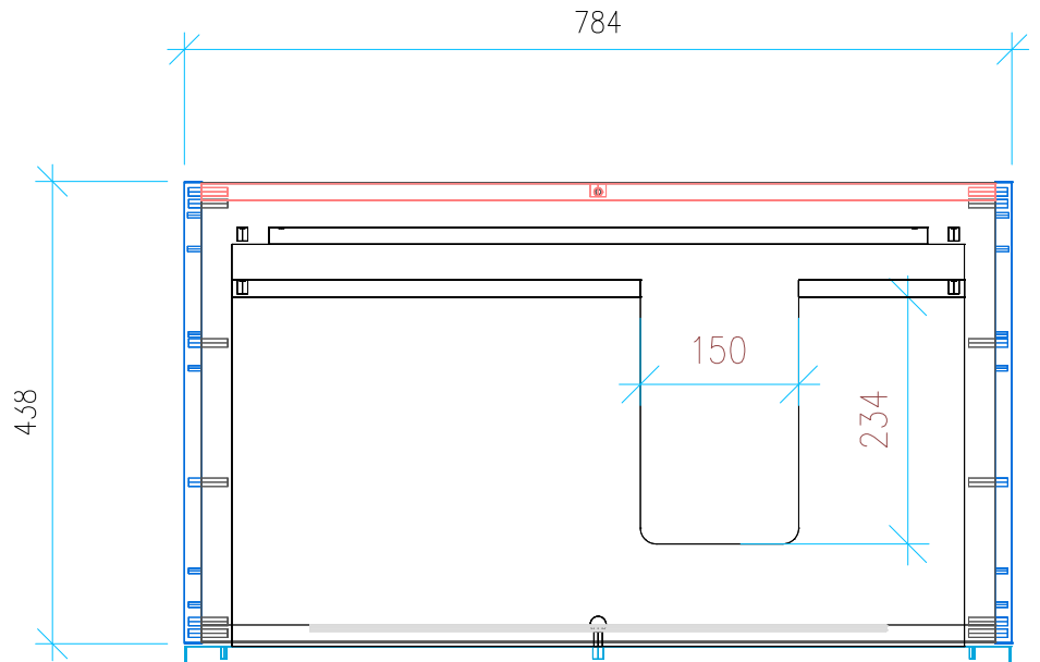
Ansicht 2 / Draufsicht
