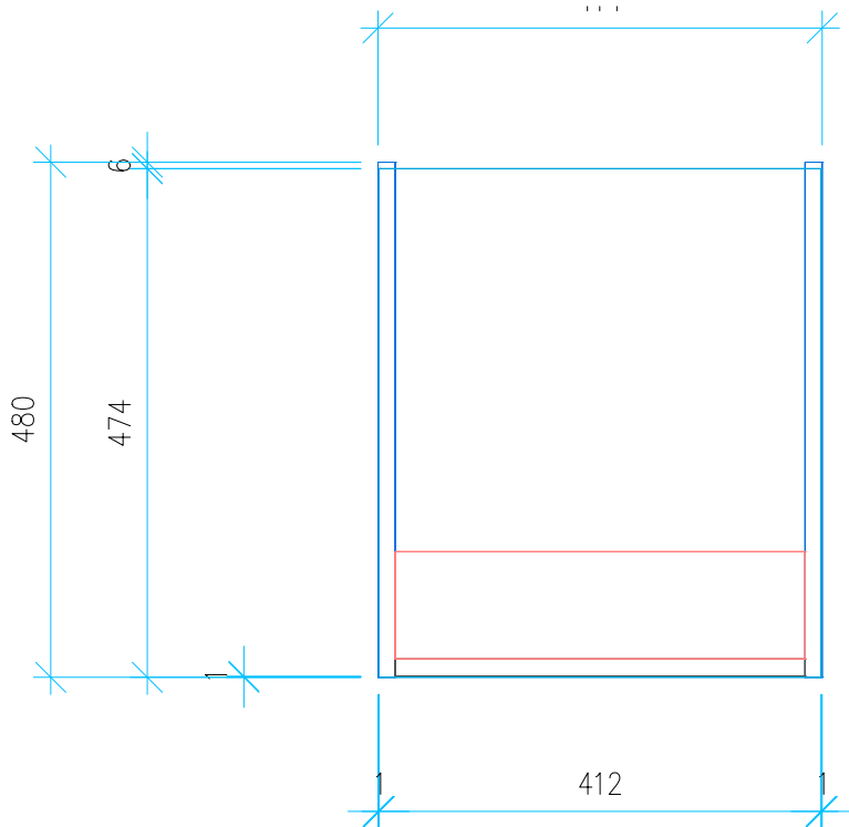
Ansicht 4 / Vorderansicht
