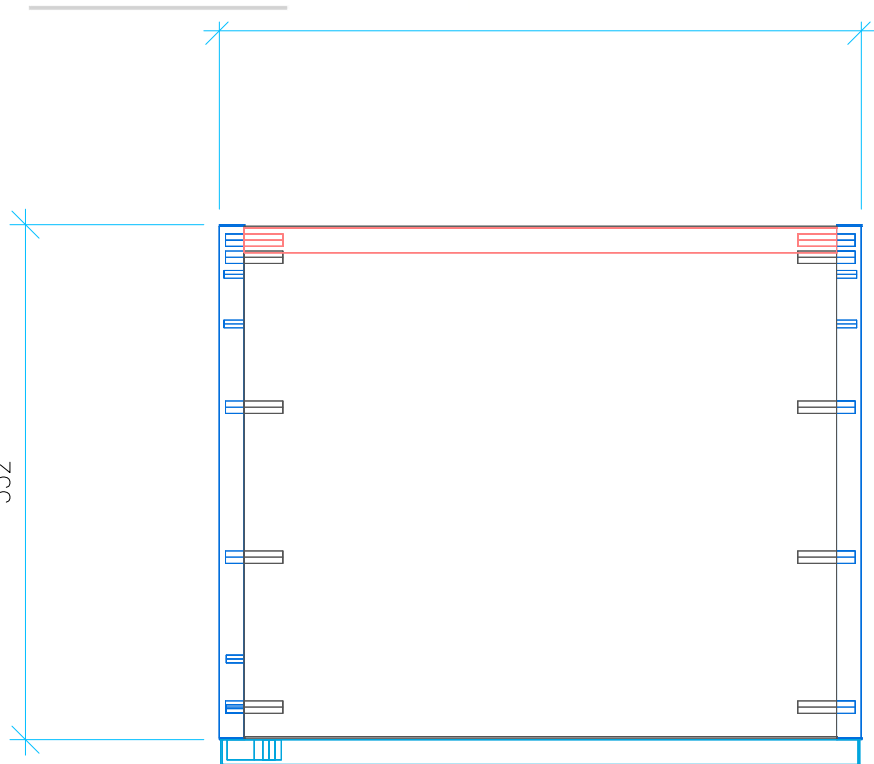
Ansicht 2 / Draufsicht
