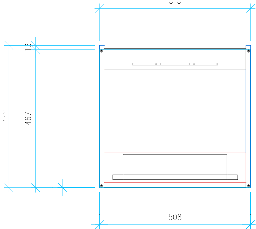
Ansicht 4 / Vorderansicht
