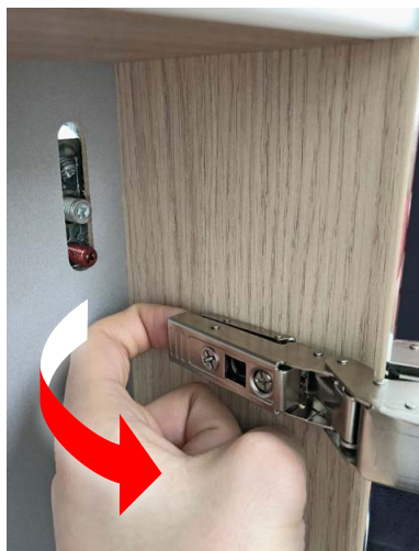
Abb. 1a | Demontage
