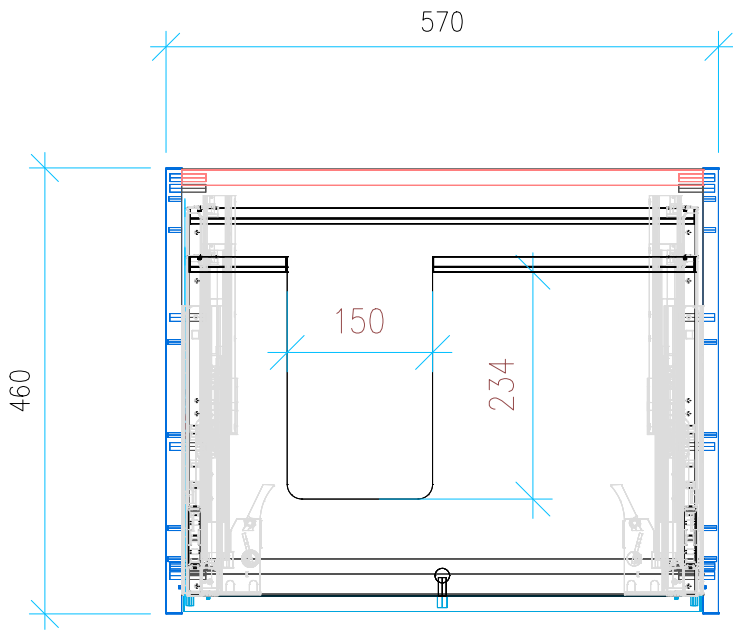
Ansicht 2 / Draufsicht
