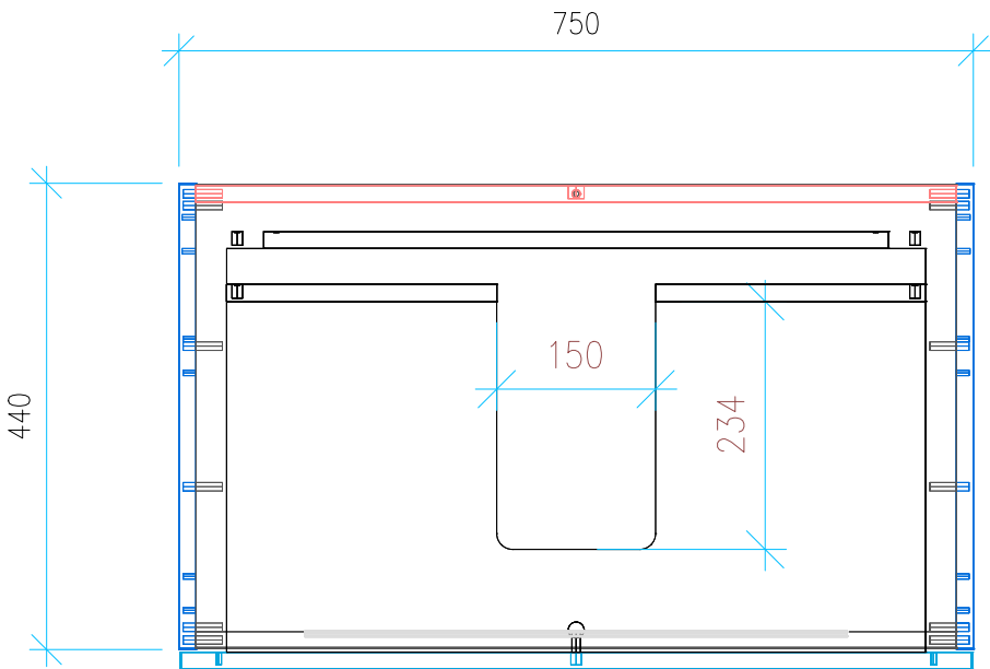
Ansicht 2 / Draufsicht
