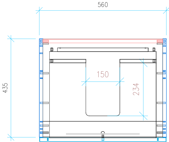
Ansicht 2 / Draufsicht
