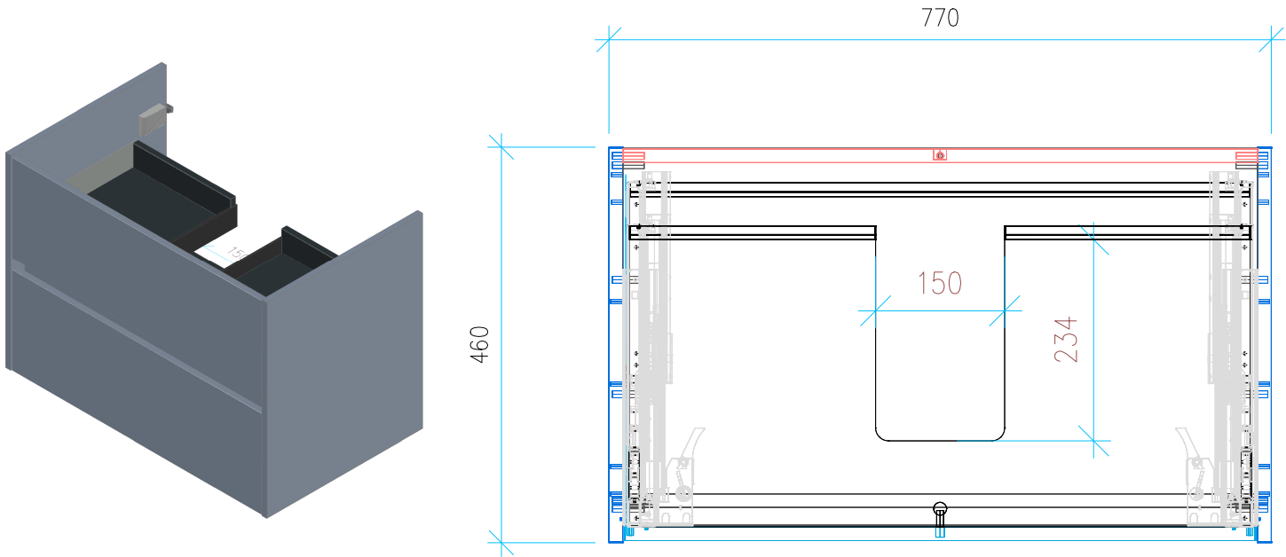
Ansicht 1 / 3D
