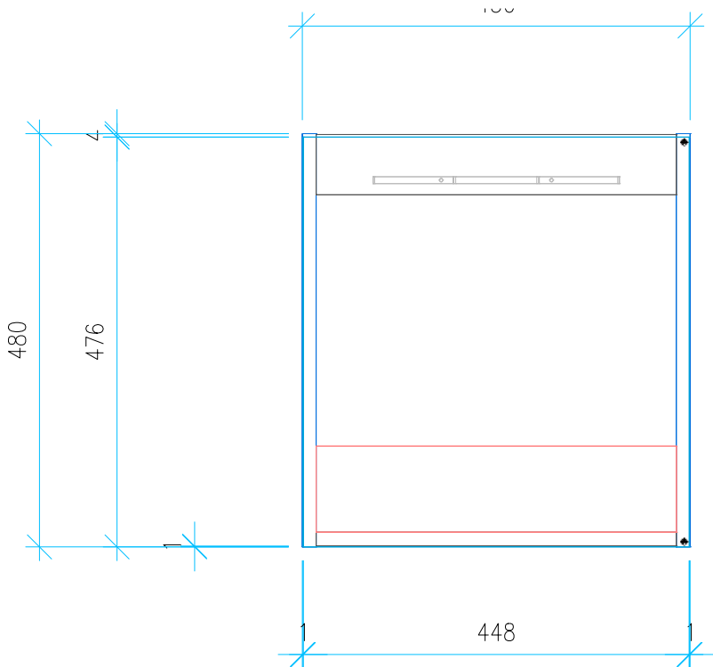
Ansicht 4 / Vorderansicht
