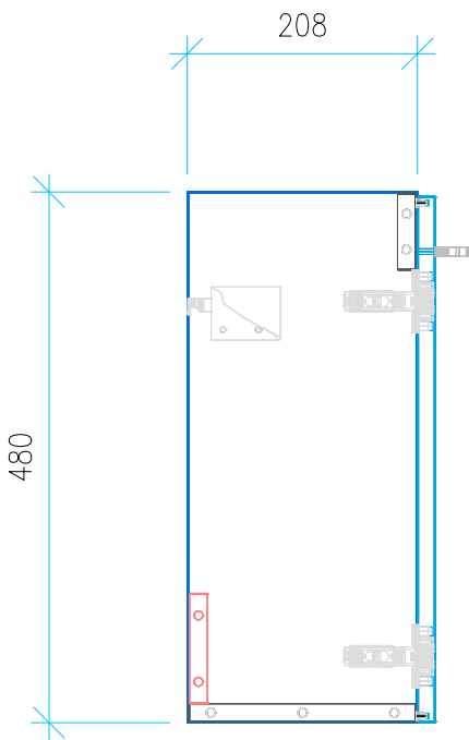
Ansicht 3 / Seitenansicht Links
