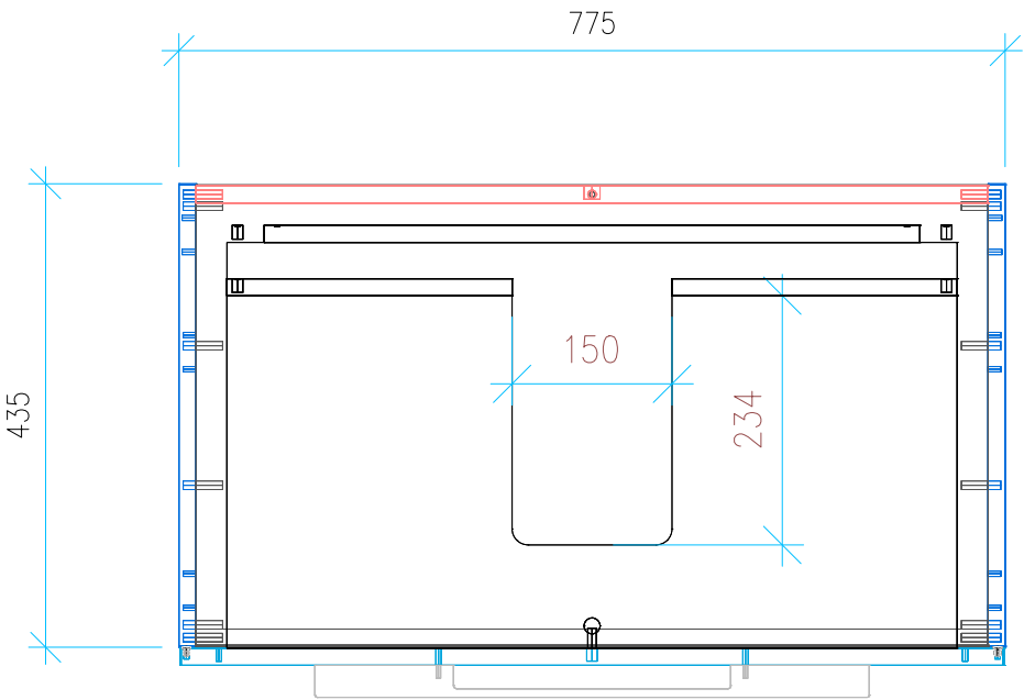
Ansicht 2 / Draufsicht
