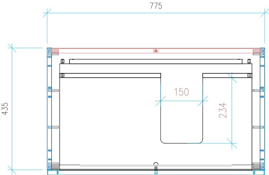
Ansicht 2 / Draufsicht
