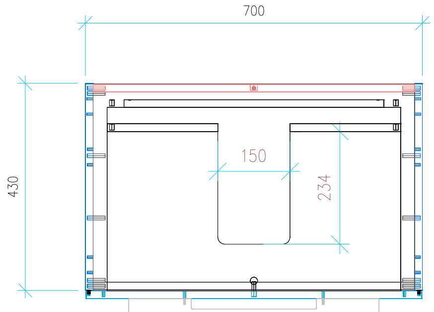
Ansicht 2 / Draufsicht
