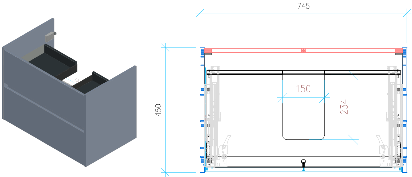
Ansicht 1 / 3D
