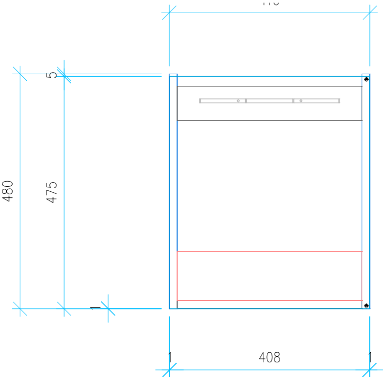
Ansicht 4 / Vorderansicht
