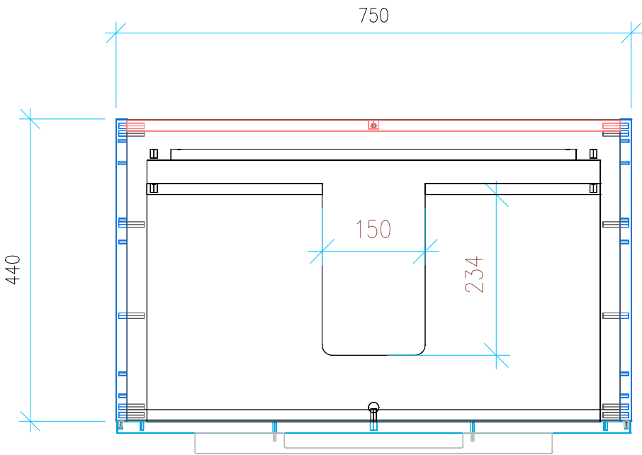
Ansicht 2 / Draufsicht
