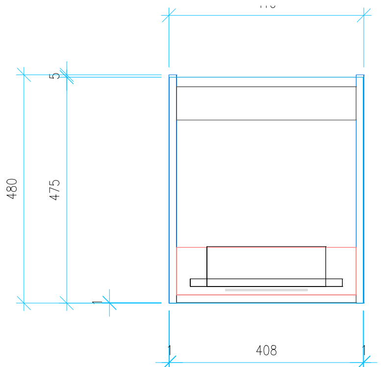
Ansicht 4 / Vorderansicht
