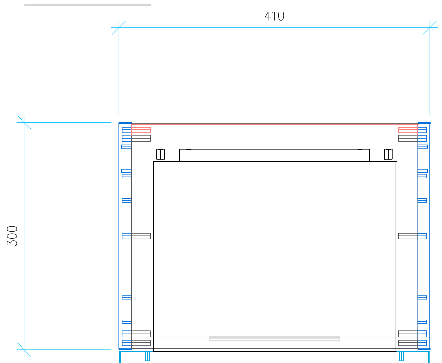
Ansicht 2 / Draufsicht
