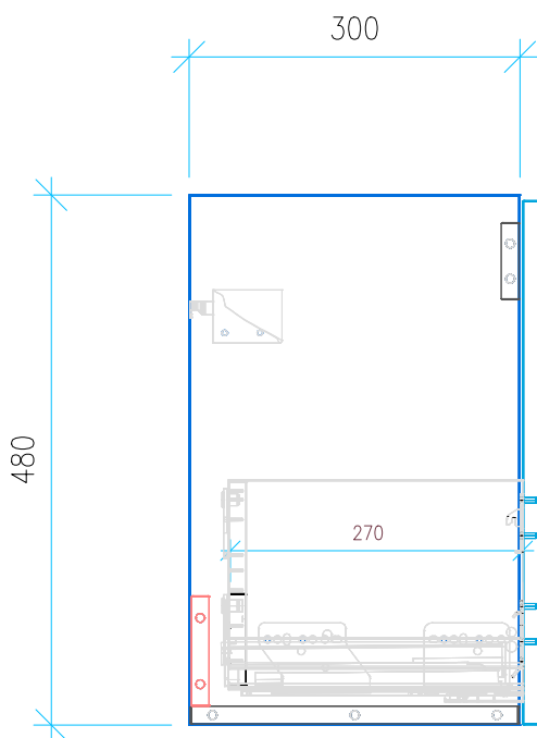
Ansicht 3 / Seitenansicht Links
