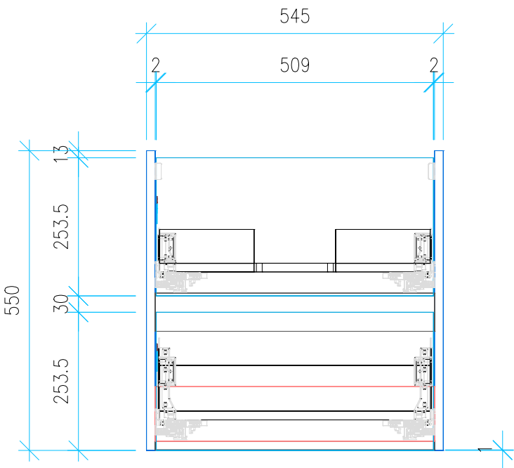
Ansicht 4 / Vorderansicht
