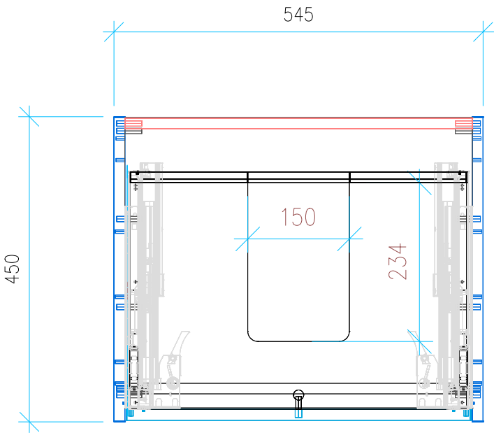
Ansicht 2 / Draufsicht
