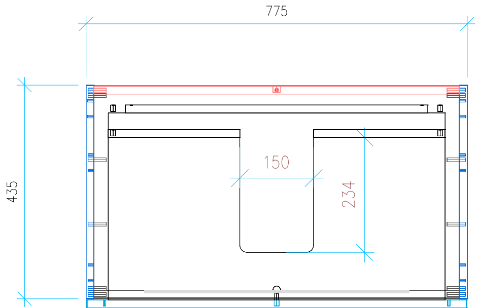
Ansicht 2 / Draufsicht
