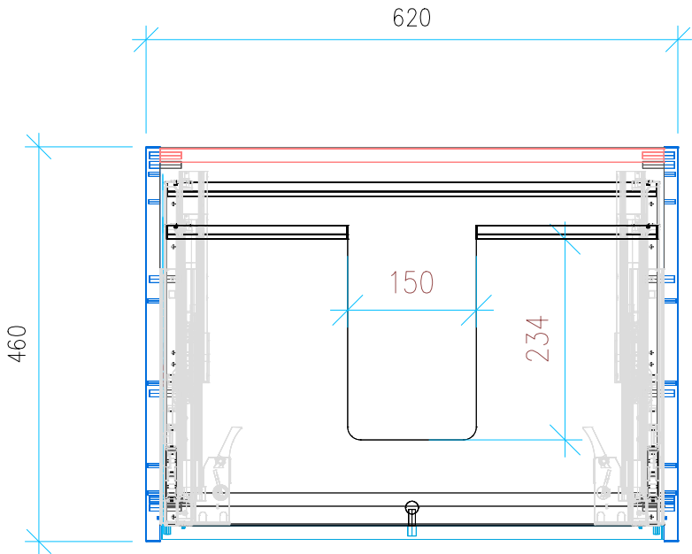
Ansicht 2 / Draufsicht
