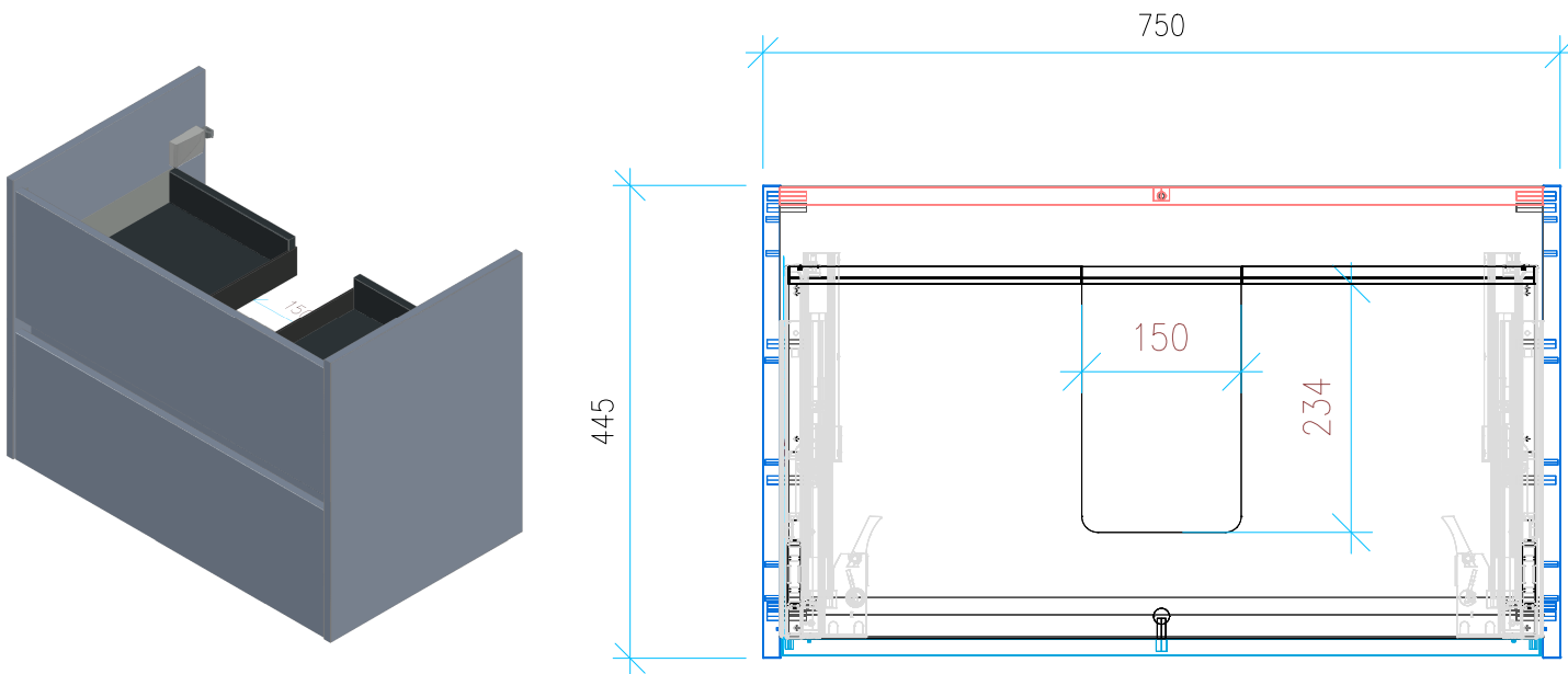
Ansicht 1 / 3D
