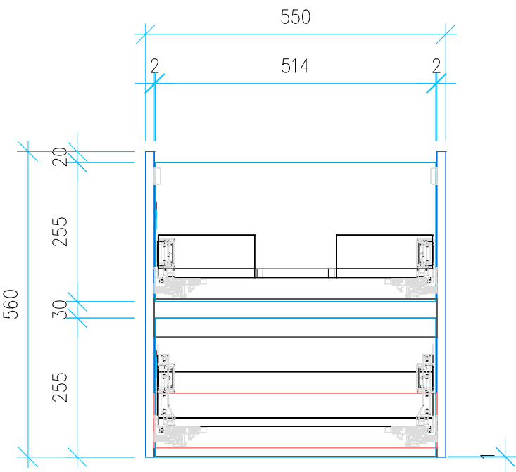
Ansicht 4 / Vorderansicht
