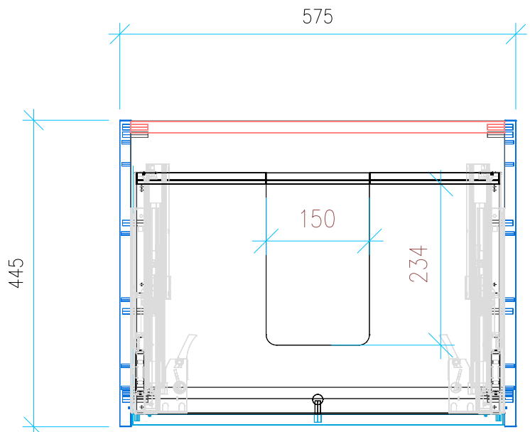
Ansicht 2 / Draufsicht
