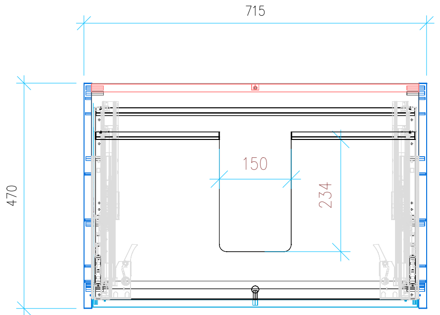
Ansicht 2 / Draufsicht
