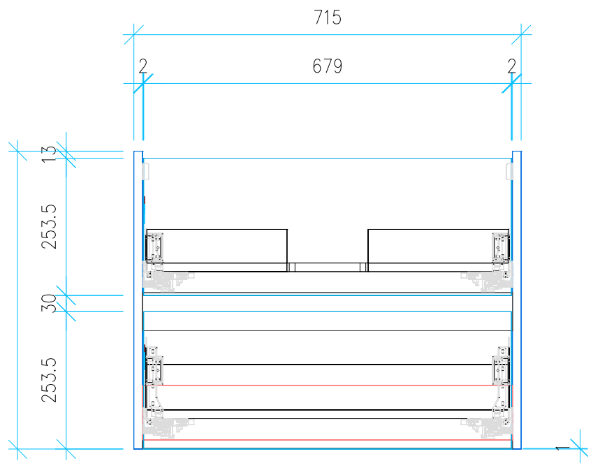
Ansicht 4 / Vorderansicht
