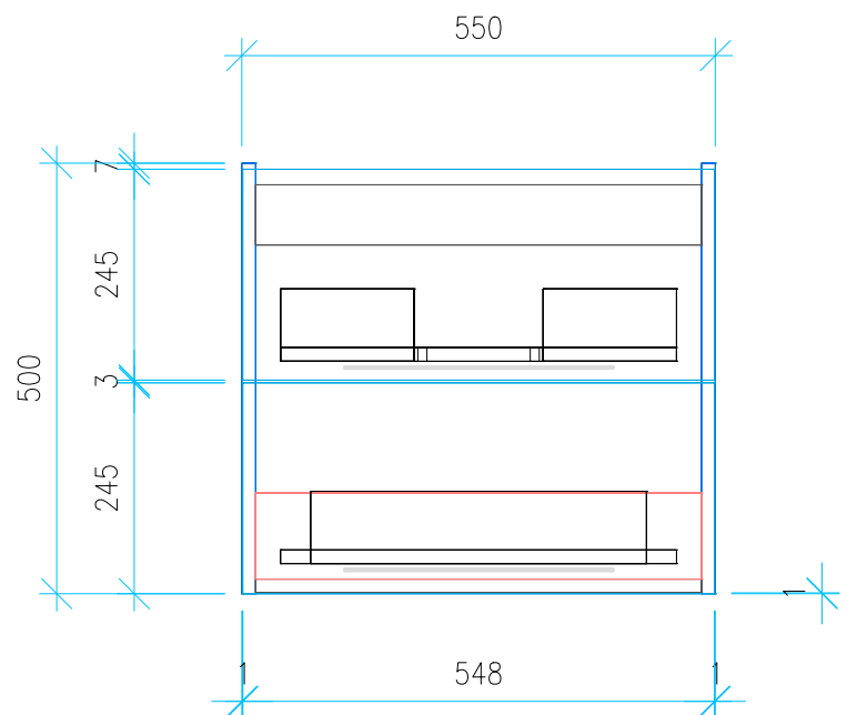
Ansicht 4 / Vorderansicht
