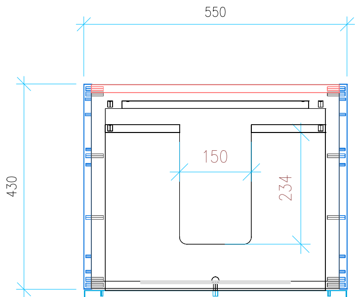
Ansicht 2 / Draufsicht
