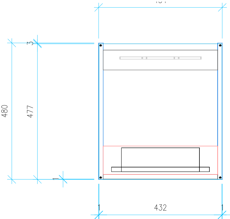
Ansicht 4 / Vorderansicht
