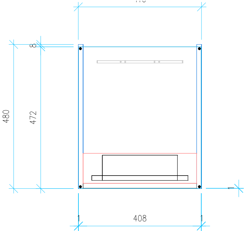
Ansicht 4 / Vorderansicht
