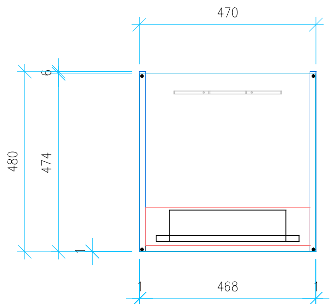
Ansicht 4 / Vorderansicht
