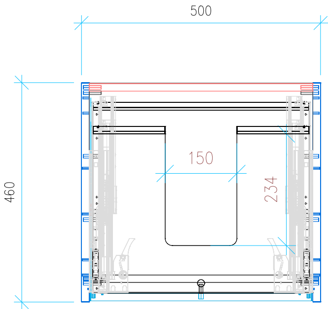
Ansicht 2 / Draufsicht
