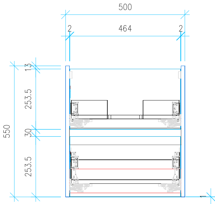
Ansicht 4 / Vorderansicht
