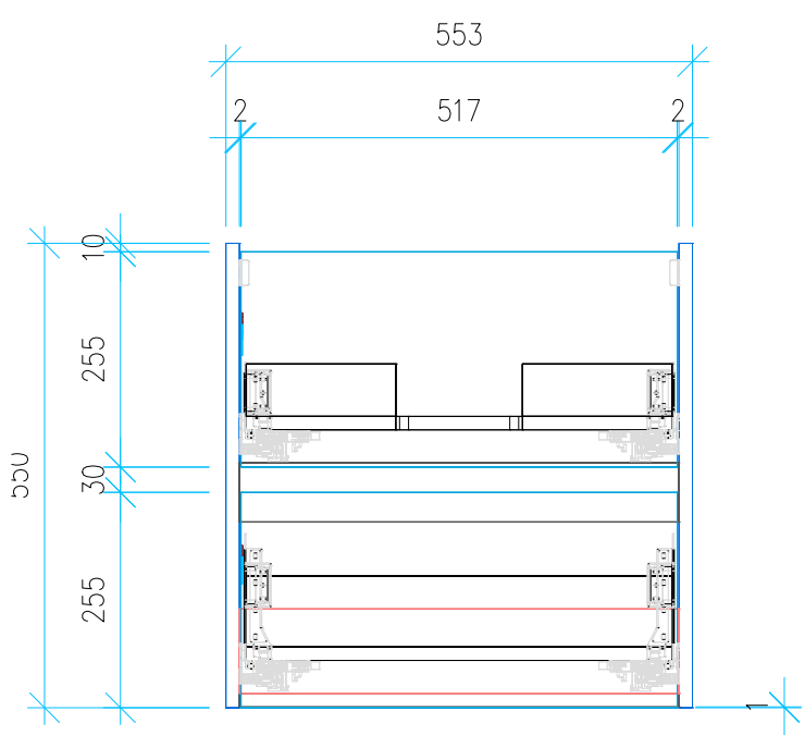
Ansicht 4 / Vorderansicht
