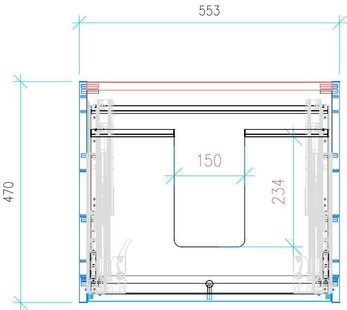
Ansicht 2 / Draufsicht
