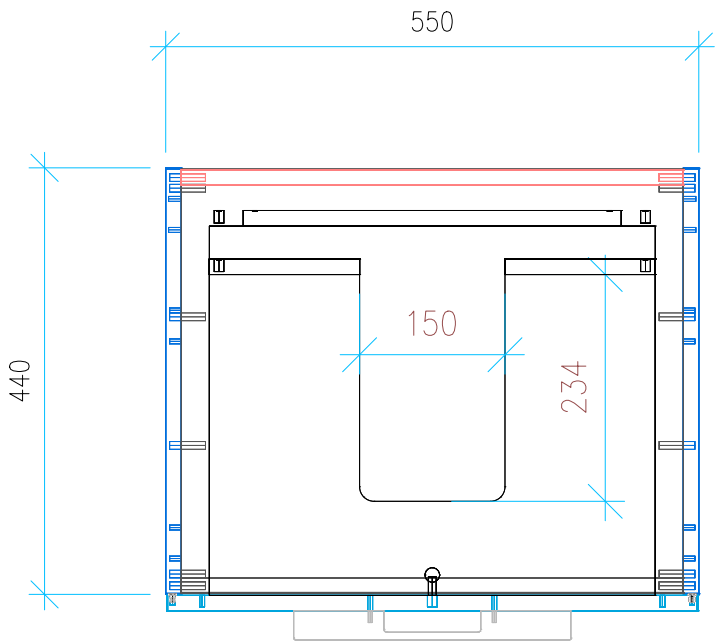
Ansicht 2 / Draufsicht
