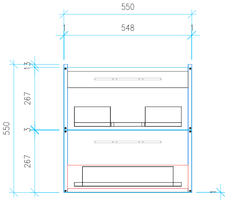
Ansicht 4 / Vorderansicht
